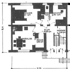
ZWEIFAMILIENWOHNHAUS ERD- UND OBERGESCHOSS
